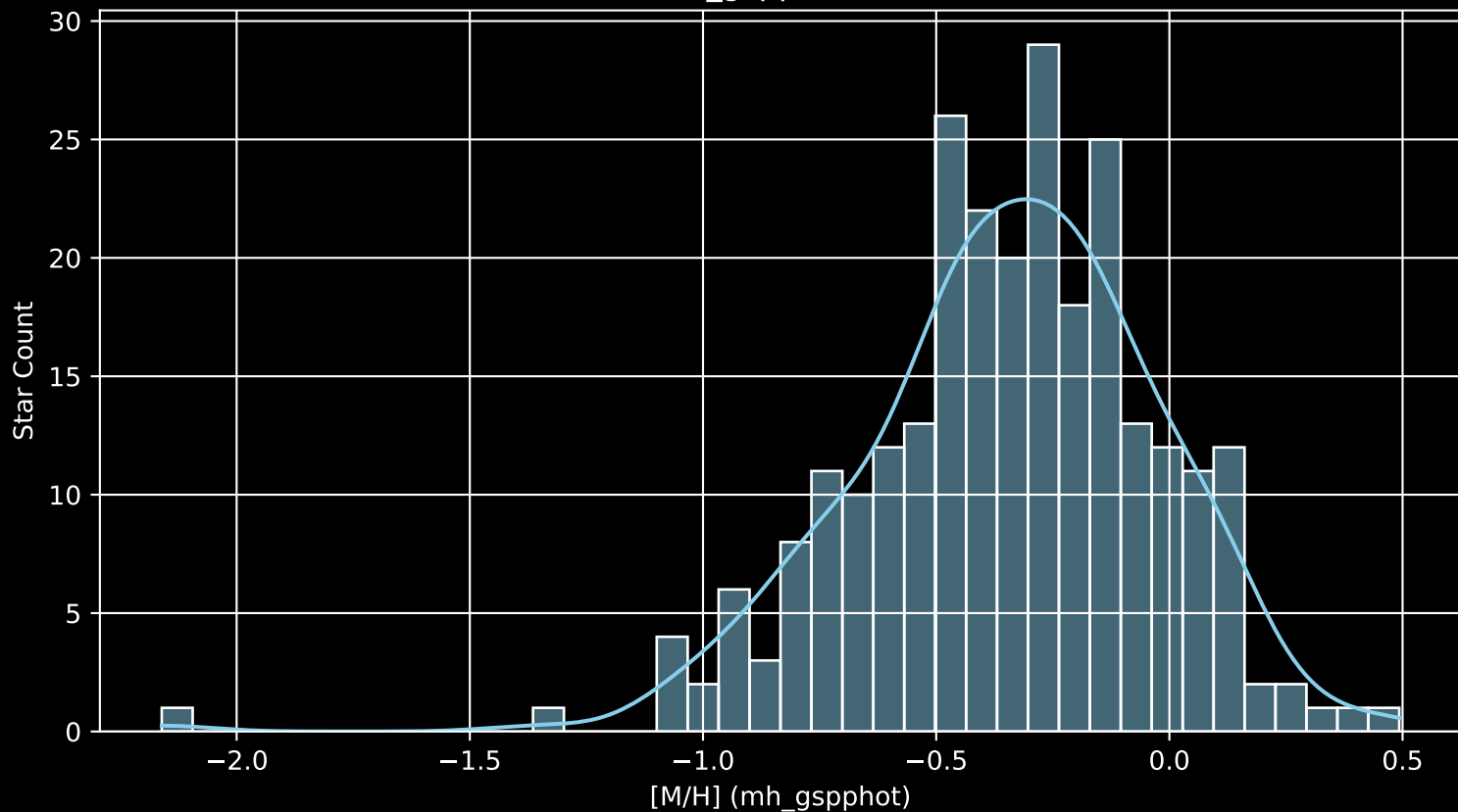
GALAH DR4 Field: [1646] [M/H] (mh_gspphot) (n= 266)
