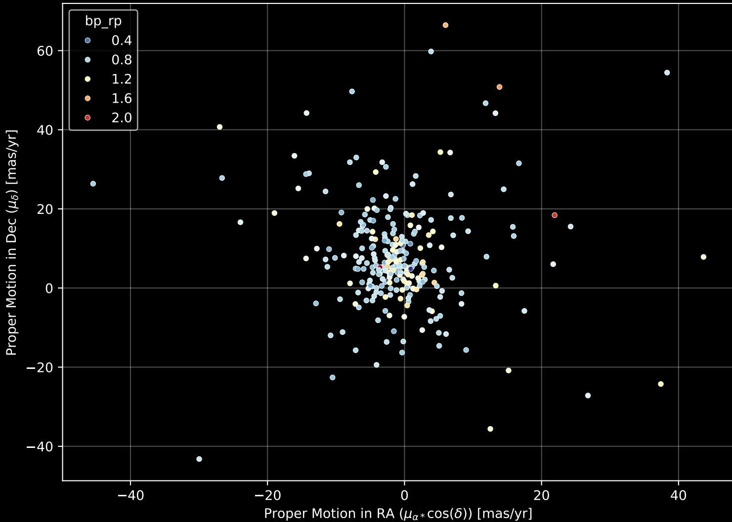
GALAH DR4 Field: [1646] Proper Motion Diagram (n= 266)
