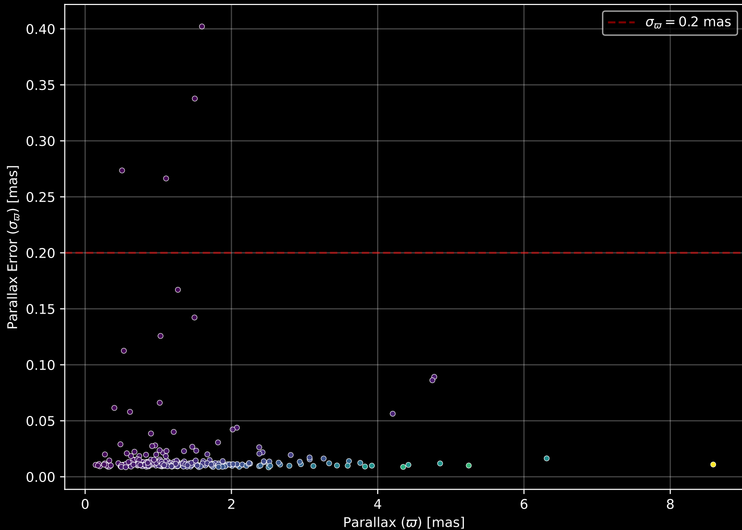
GALAH DR4 Field: [1646] Parallax Quality (n= 266)
