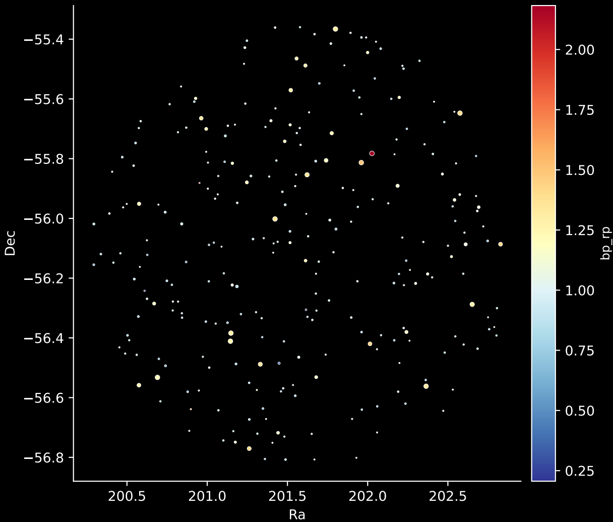
GALAH DR4 Field: [1646] Stars: 266
