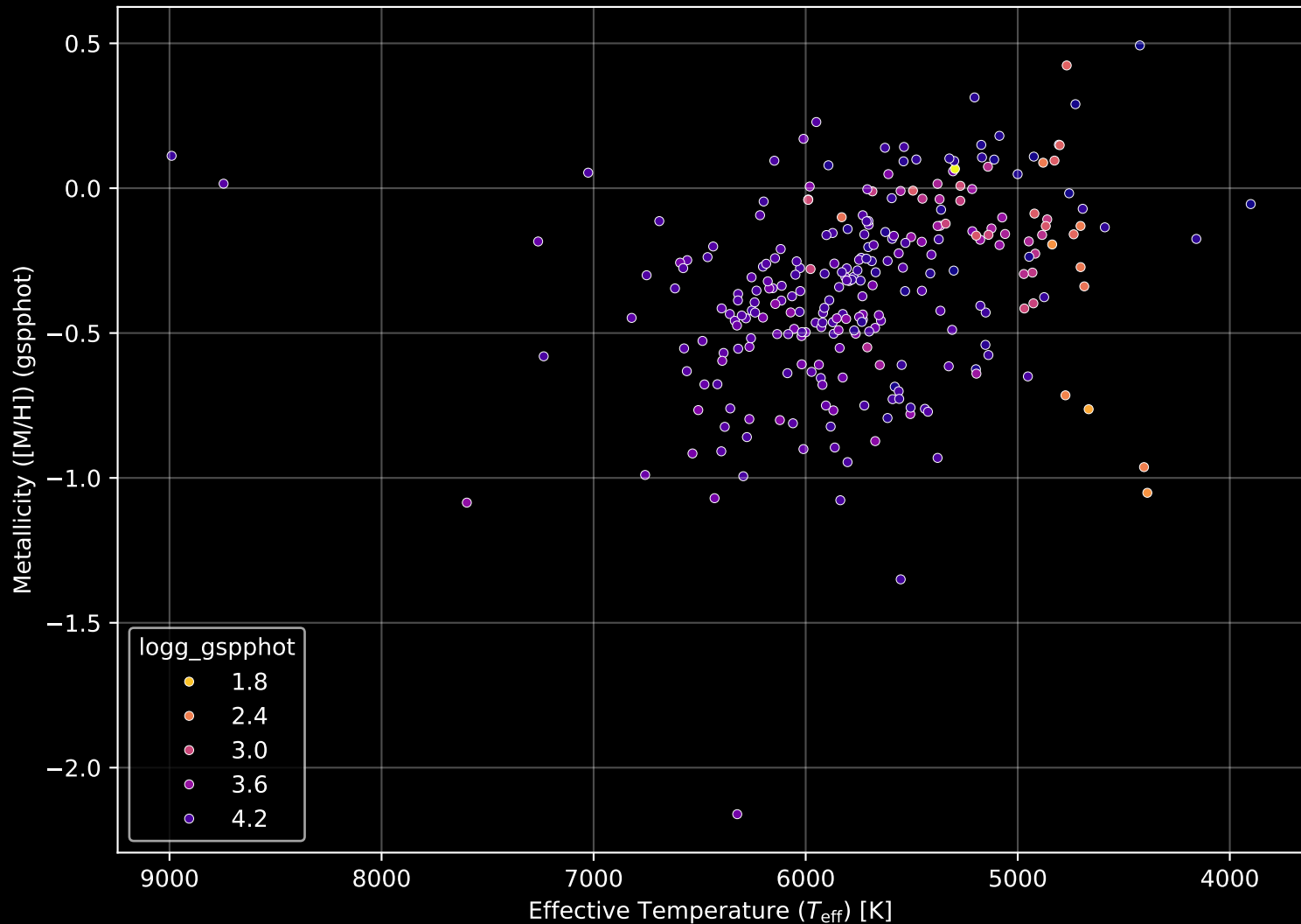
GALAH DR4 Field: [1646] Stellar Population Parameters (n= 266)
